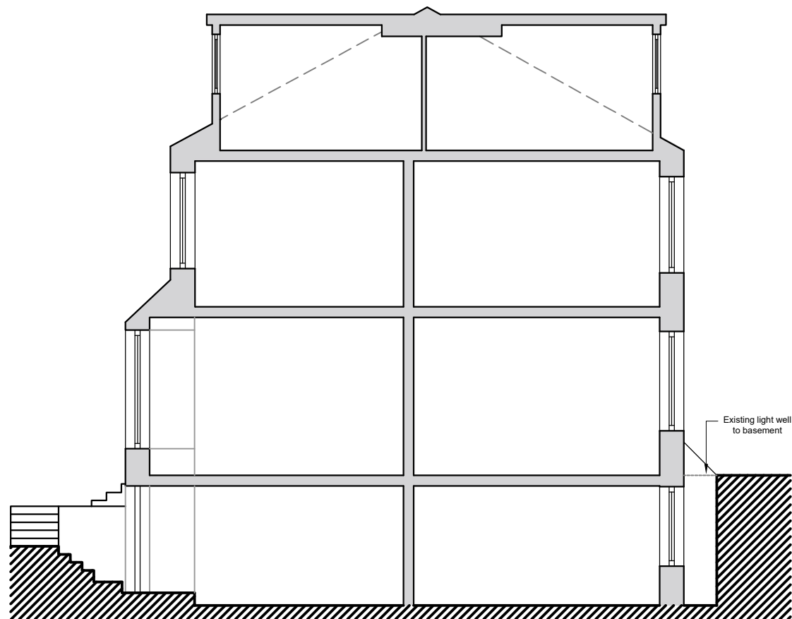
EXISTING SECTION A 1:100 @ A3
